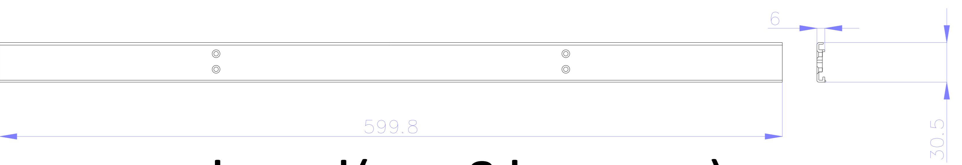
bezel(top&bottom)
